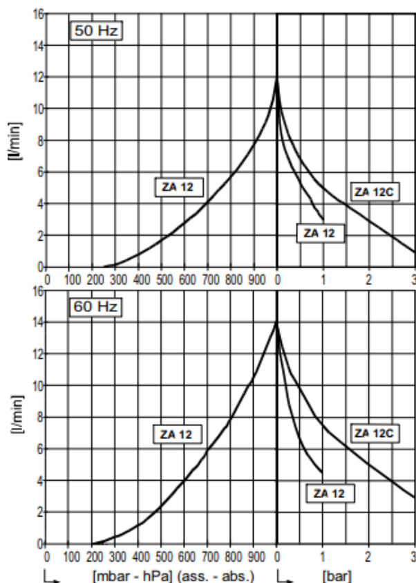
NOTA: Curve riferite alla pressione di 1013mbar (ass.) e temp. 20°C (tolleranza ±10%).
